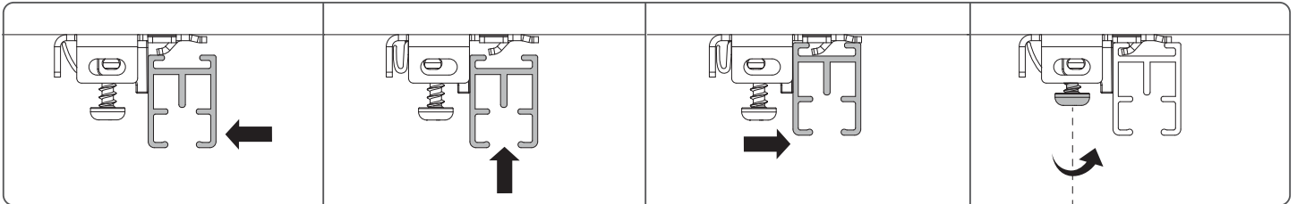
One Way Pleated - Single Panel Rideaux à plis à sens unique - Panneau unique Plisado unidireccional - Panel único
